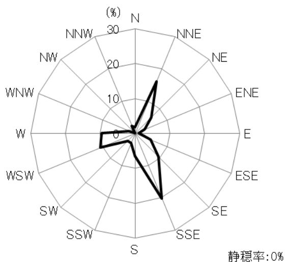
図 2-1-2 風配図
